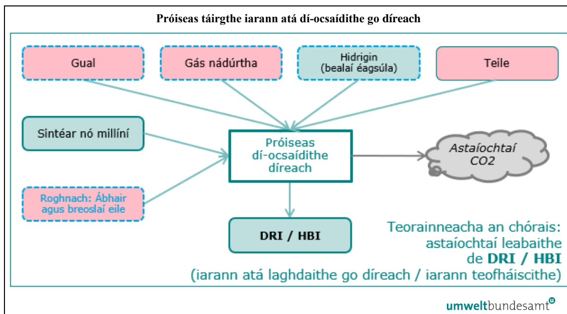
Fíor 5-10: Teorainneacha córais an phróisis táirgthe iarann atá dí-ocsaídithe go díreach
