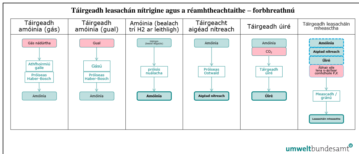
Fíor 5-4: Teorainneacha córais agus an slabhra luacha chun leasachán nítrigine agus a réamhtheachtaithe a tháirgeadh – forbhreathnú
