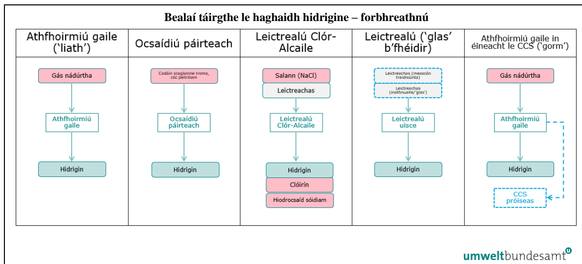
Fíor 5-3: Teorainneacha córais maidir le bealaí táirgthe difriúla le haghaidh hidrigine – forbhreathnú
