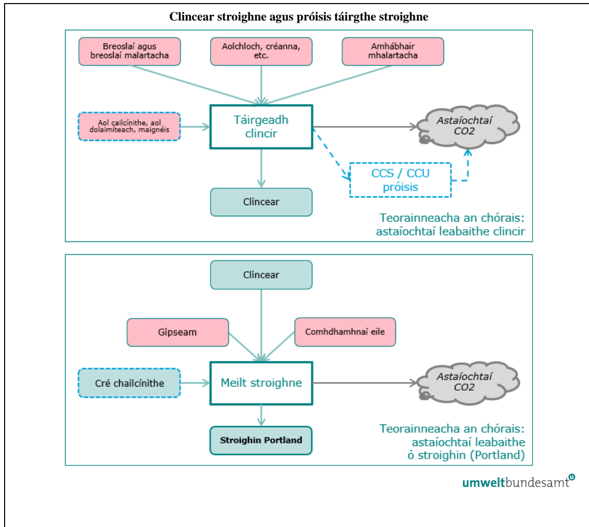
Fíor 5-1: Teorainneacha córais an chlincir stroighne agus próisis táirgthe stroighne.
