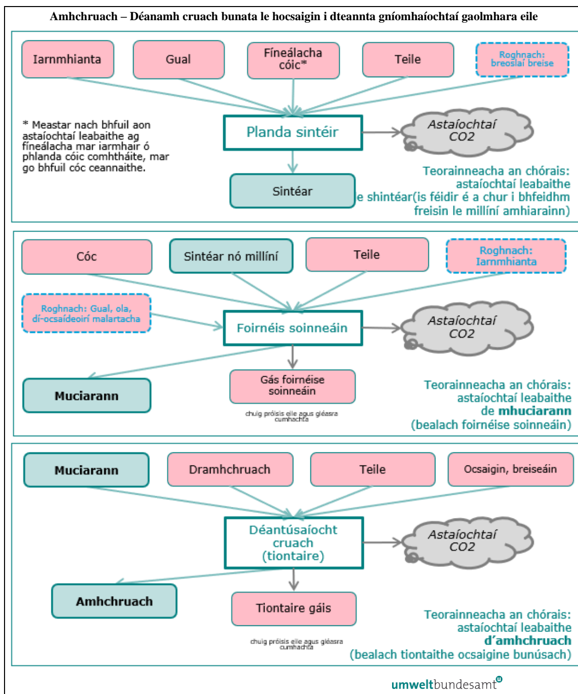
Fíor 5-11: Teorainneacha córais an phróisis déanta cruach bunata le hocsagain i dteannta gníomhaíochtaí gaolmhara eile in aice leo siúd don Fhoirnéis soinneáin – bealach táirgthe an mhuciarainn leachtaigh, agus próisis ghaolmhara eile
