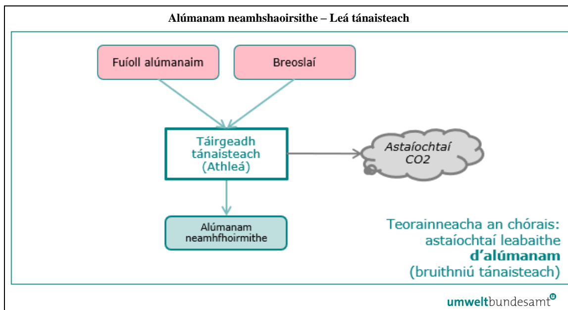
Fíor 5-16: Teorainneacha córais an alúmanaim neamhshaoirsithe - an bealach táirgthe (leictrealaíoch) tánaisteach trí bhruithniúchán
