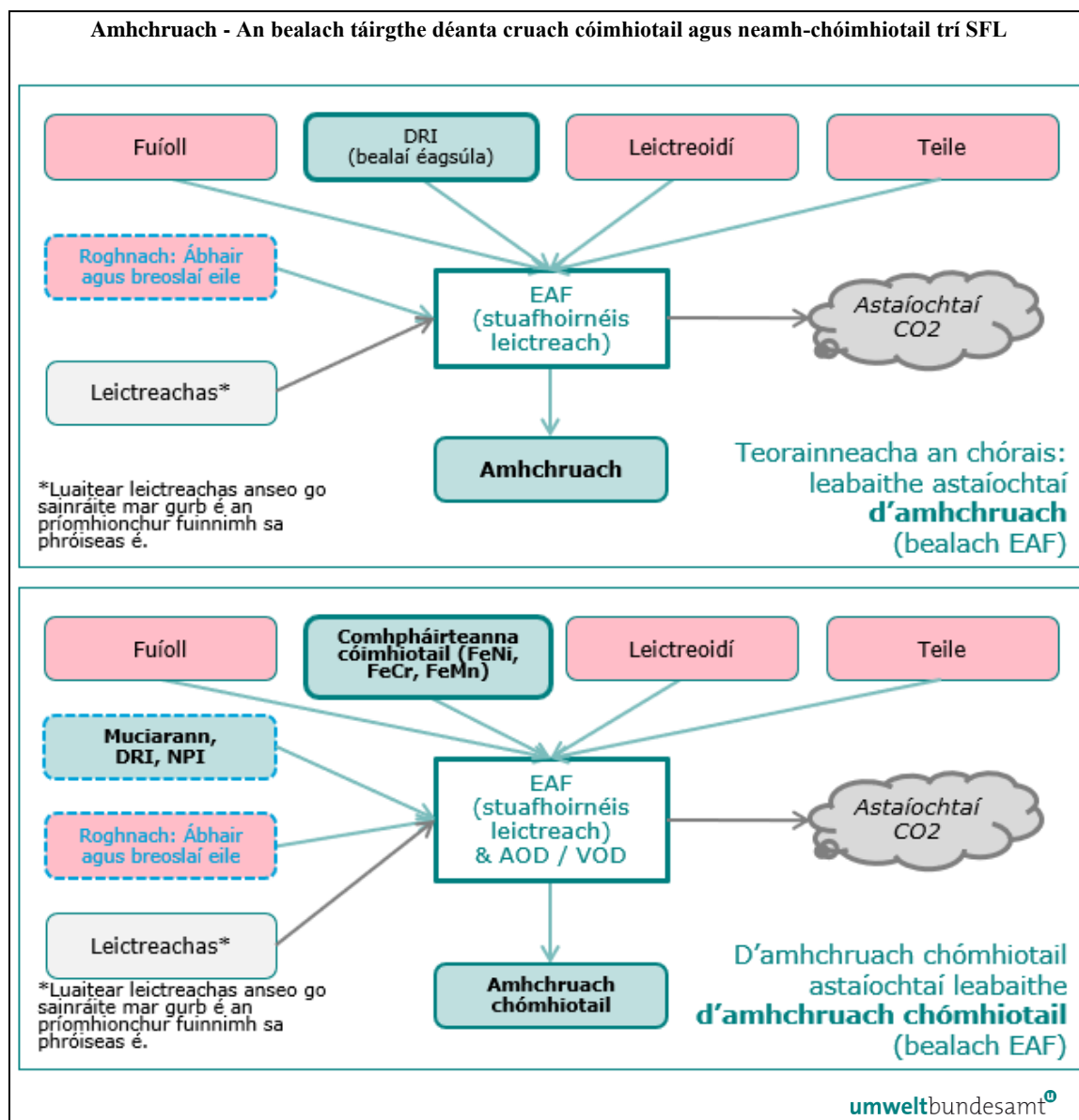
Fíor 5-12: Teorainneacha córais an bhealaigh táirgthe amhchruach - déanamh cruach trí SFL.
