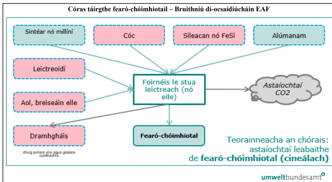
Fíor 5-7: Teorainneacha córais don phróiseas táirgthe fearó-chóimhiotail.
