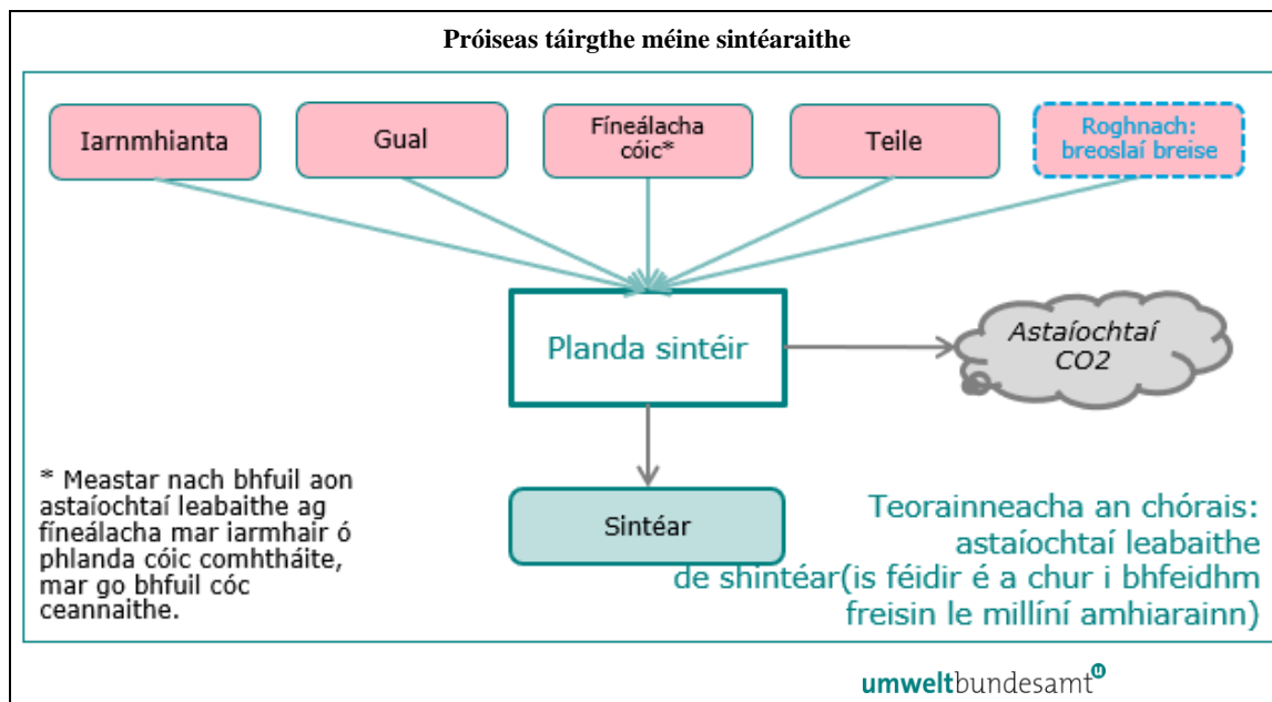
Fíor 5-6: Teorainneacha córais na bpróiseas táirgthe méine sintéaraithe
