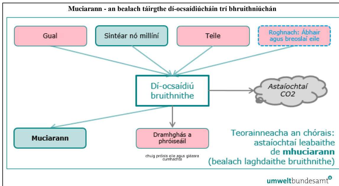
Fíor 5-9: Teorainneacha córais an mhuciarainn - an bealach táirgthe dí-ocsaídiúcháin trí bhruithniúchán
