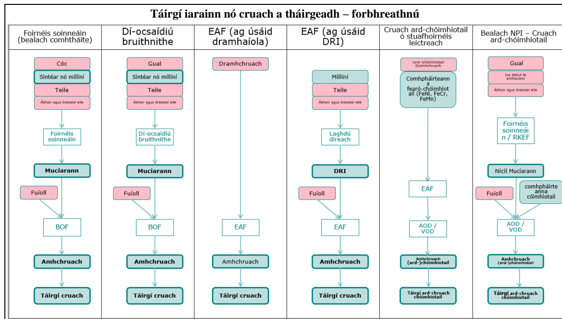
Fíor 5-5: Teorainneacha córais agus slabhra luacha le haghaidh táirgí iarainn nó cruach a tháirgeadh
